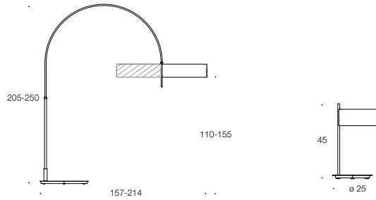
Bogenleuchte / Arc lamp BW-L-101-400
