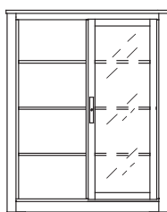
Regal mit 1 Glastür B 132 T 47 H 166 cm
