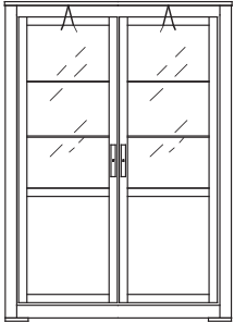
B 152 T 42 H 213 cm
