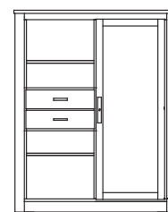
Regal mit Holztür und Schubkästen B 132 T 47 H 166 cm
